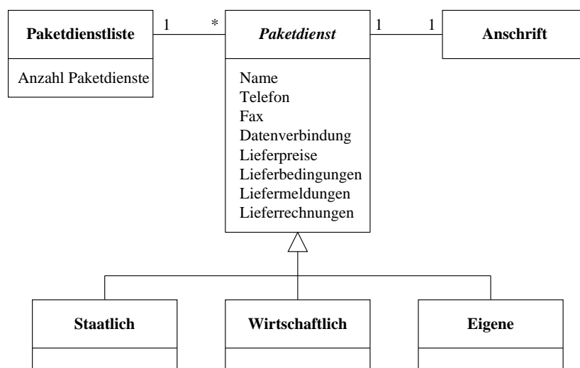
Abbildung 4.18: Fachklassendiagramm zu den Paketdiensten
