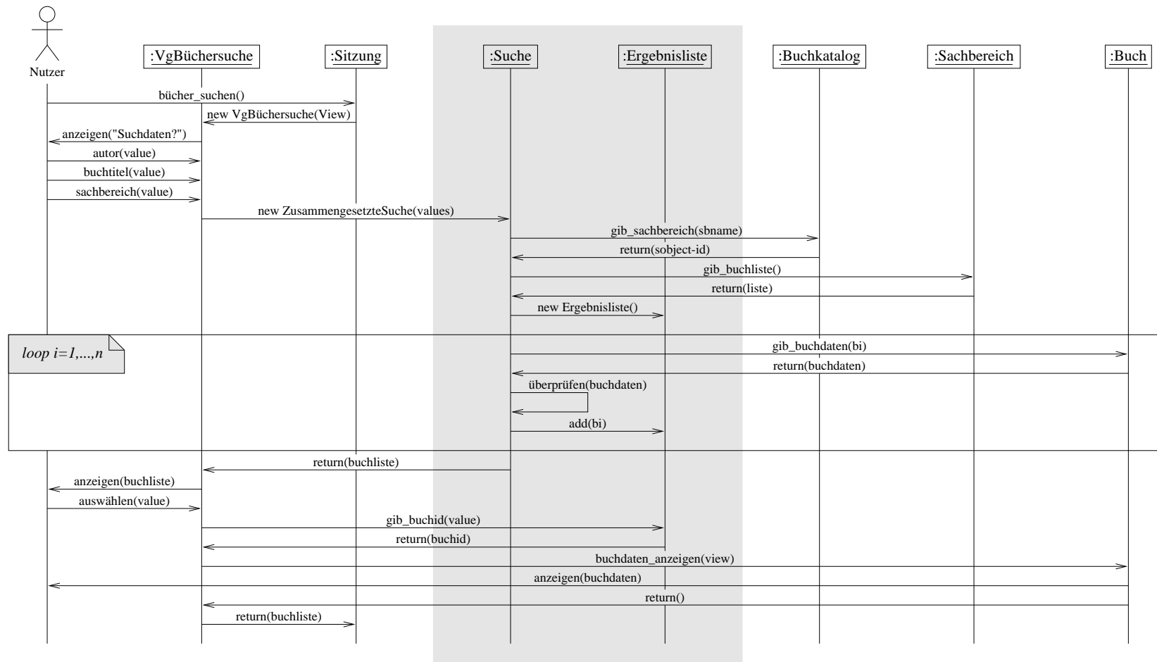
Abbildung 6.28: Erweitertes Sequenzdiagramm zum Nutzungsfall Büchersuche
