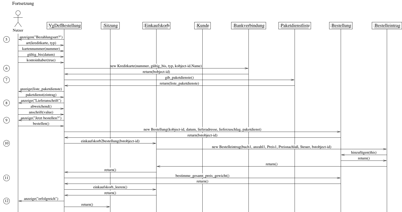
Abbildung 6.11: Sequenzdiagramm zum Nutzungsfall: Bestellung der im Einkaufskorb liegenden Bücher (Teil 2)
