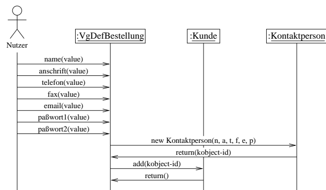
Abbildung 6.19: Teil-Sequenzdiagramme zum HMSC: korb- und kundendaten
