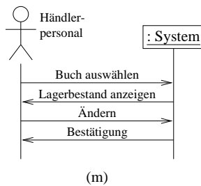
Abbildung 5.8: Bestellverwaltung als Funktion der Händler-Sitzung (Teil 2)
