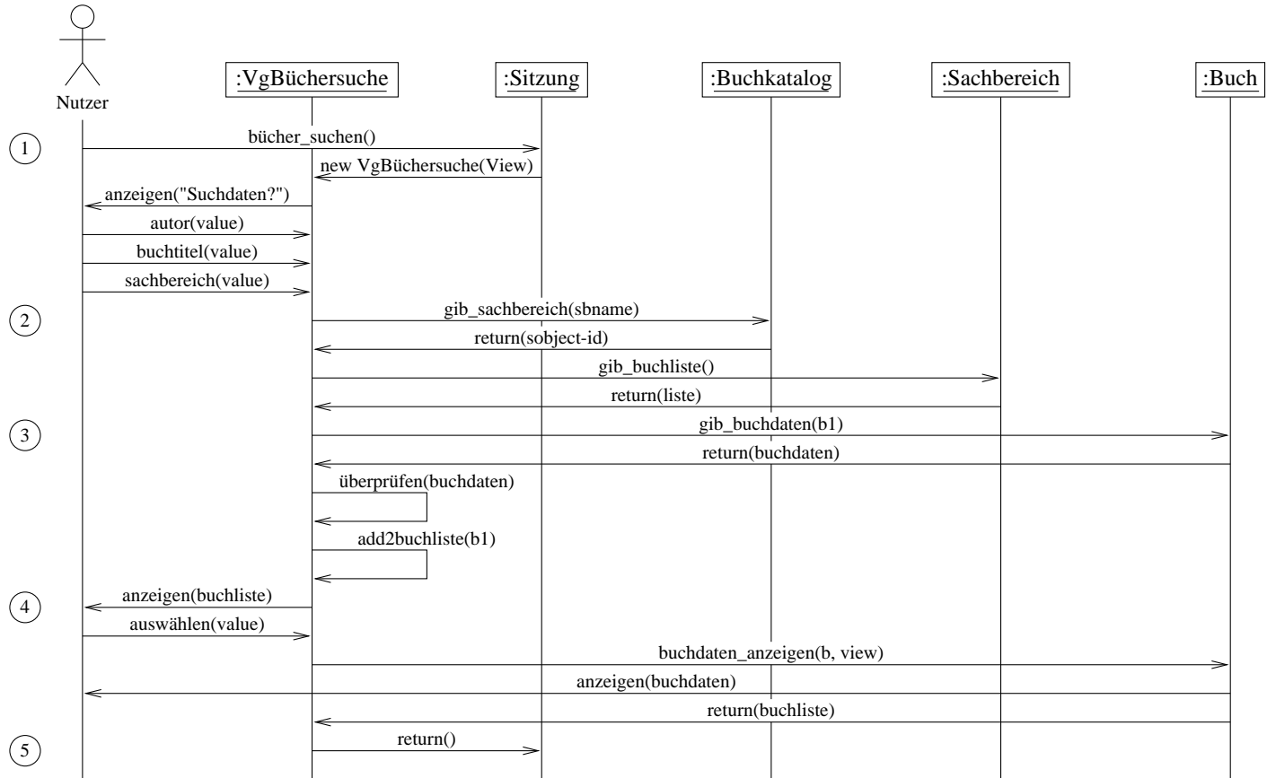
Abbildung 6.27: Sequenzdiagramm zum Nutzungsfall: Büchersuche
