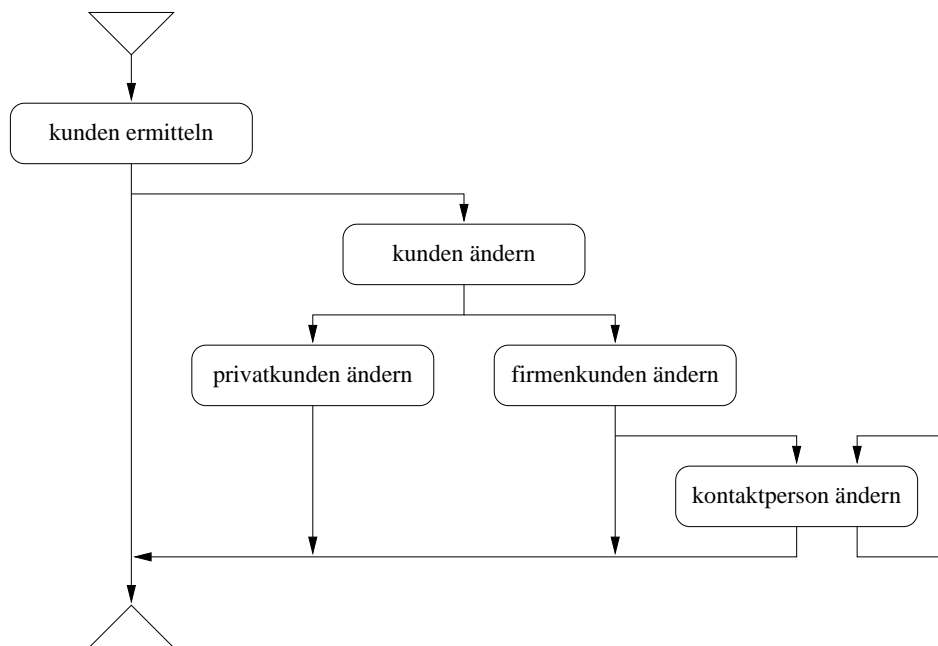
Abbildung 6.20: HMSC zur Ermittlung und Bearbeitung von Kundendaten bei einer wiederholten Bestellung
