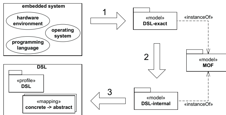
Abbildung 1: Erstellung einer DSL auf Basis von MOF und UML
