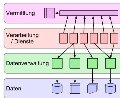
Abbildung 1: Strukturelle Architektur einer Leitsteuerung
