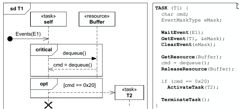
Abbildung 10: Verhalten von Task T1 (Sequenzdiagramm und C Code)
