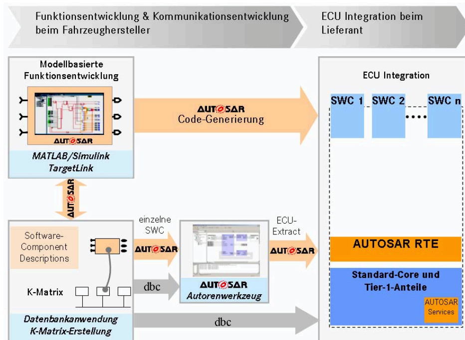
Abbildung 3: AUTOSAR-Werkzeugumgebung
